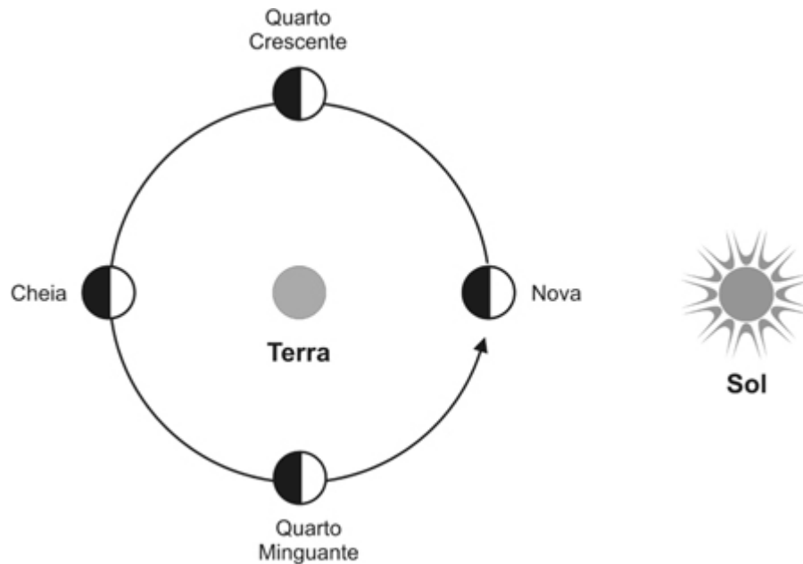
Fases da Lua.
