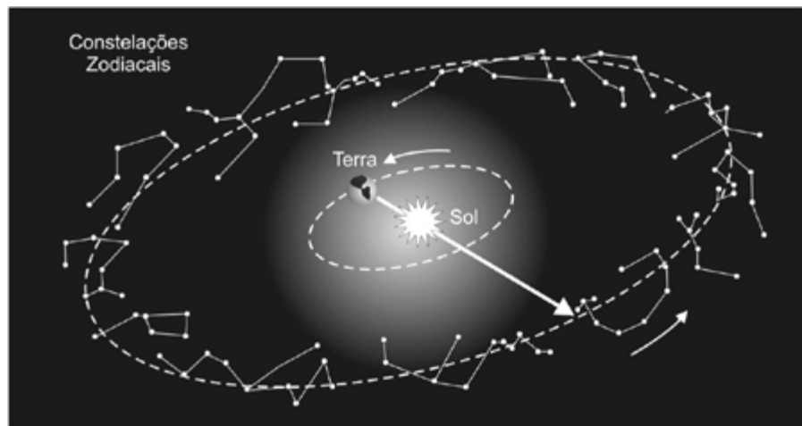
Movimento aparente do Sol na Eclíptica.
