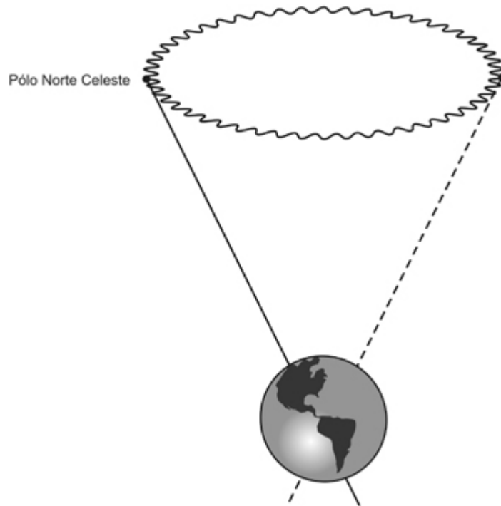
Nutação e precessão da Terra.
