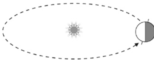
Órbita da Terra ao redor do Sol com eixo de rotação da Terra.
