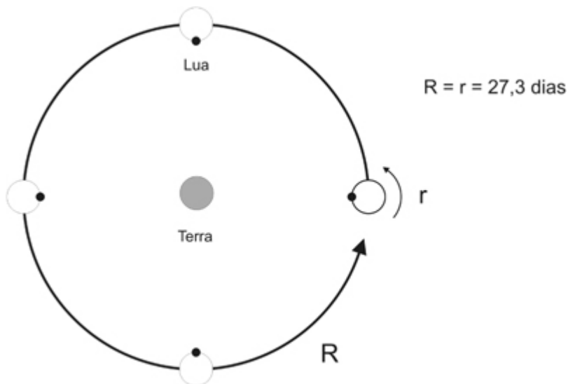
Movimento síncrono da Lua.
