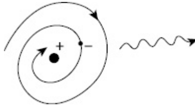
FIGURA 5.11 Instabilidade do modelo atômico de Rutherford.
