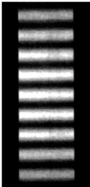
FIGURA 5.7 Um padrão de interferência formado por luz passando através de duas fendas estreitas.
