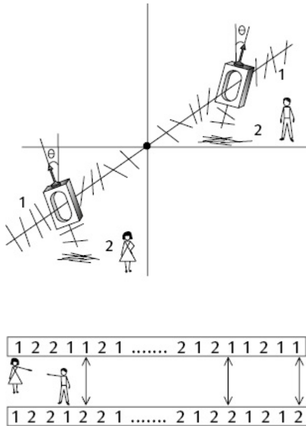
FIGURA 13.5 Experimento IV: Os polarizadores de Alice e Bob são ambos girados e as descombinações se devem a ambas as rotações.
