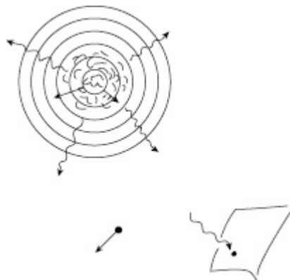
FIGURA 10.3 O ricocheteamento de um fóton num átomo não cria a posição do átomo até que o fóton seja detectado.
