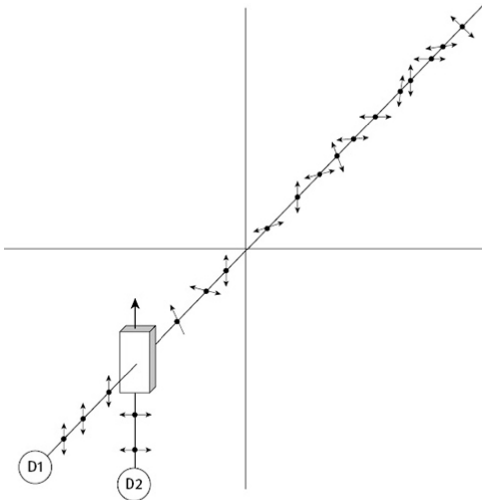
FIGURA 12.7 Fótons polarizados aleatoriamente ordenados por um polarizador.
