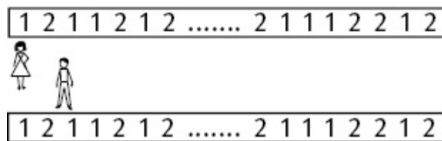
FIGURA 13.3 Experimento I: os polarizadores estão alinhados e os dados de Alice e Bob são idênticos.
