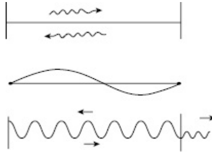
FIGURA 9.1 No alto : Ondas de luz refletidas de um lado a outro entre dois espelhos. Centro : Uma corda de violão ressoando. Embaixo : Uma onda de luz ressoando entre dois espelhos de laser.
