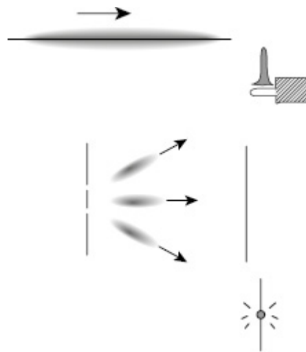
FIGURA 6.6 No alto : Ondulatoriedade de uma partícula alfa antes e depois de ser detectada por um contador Geiger. Embaixo : Ondulatoriedade de um único elétron antes e depois de ser detectado numa tela.
