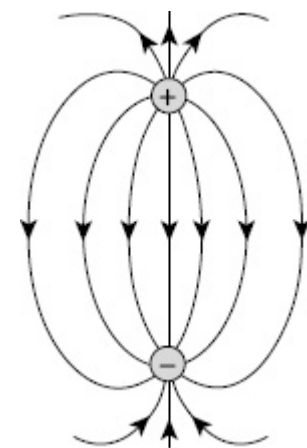
FIGURA 4.5 Campo elétrico em volta de duas cargas.
