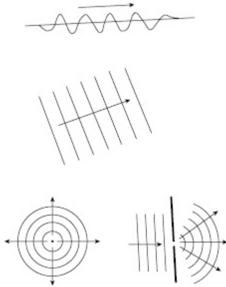
FIGURA 4.1 Imagens de ondas.
