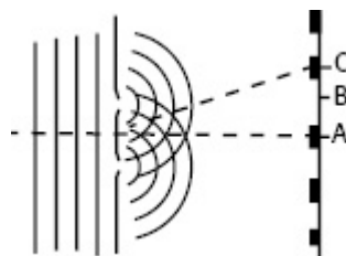
FIGURA 4.2 Interferência no experimento da dupla fenda.
