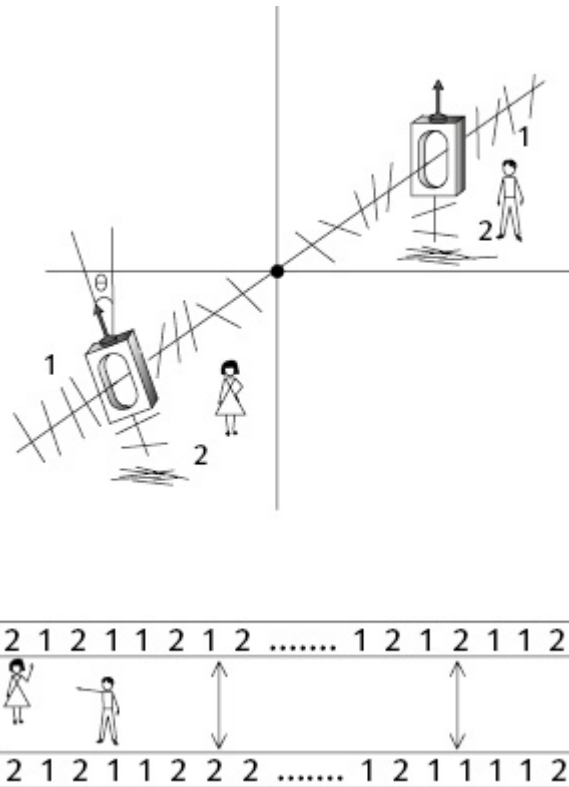
FIGURA 13.4 Experimento II: o polarizador de Alice é girado, provocando falta de concordância.
