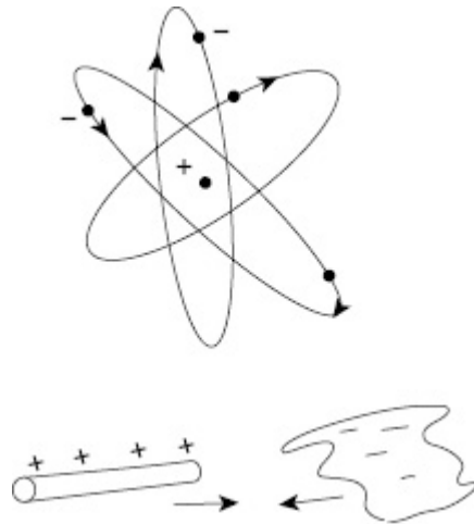
FIGURA 4.3 Cargas positivas e negativas.
