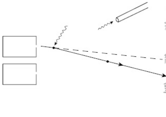
FIGURA 10.4 O microscópio de Heisenberg.
