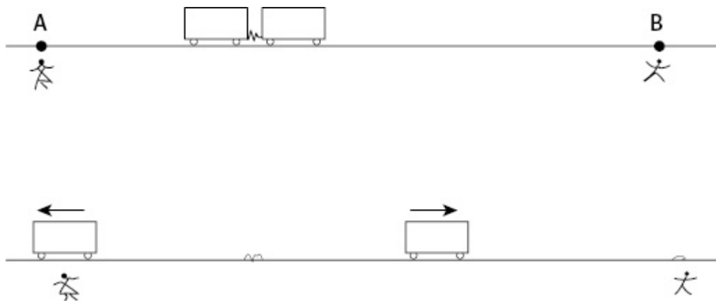
FIGURA 12.4 Uma analogia clássica do argumento EPR.
