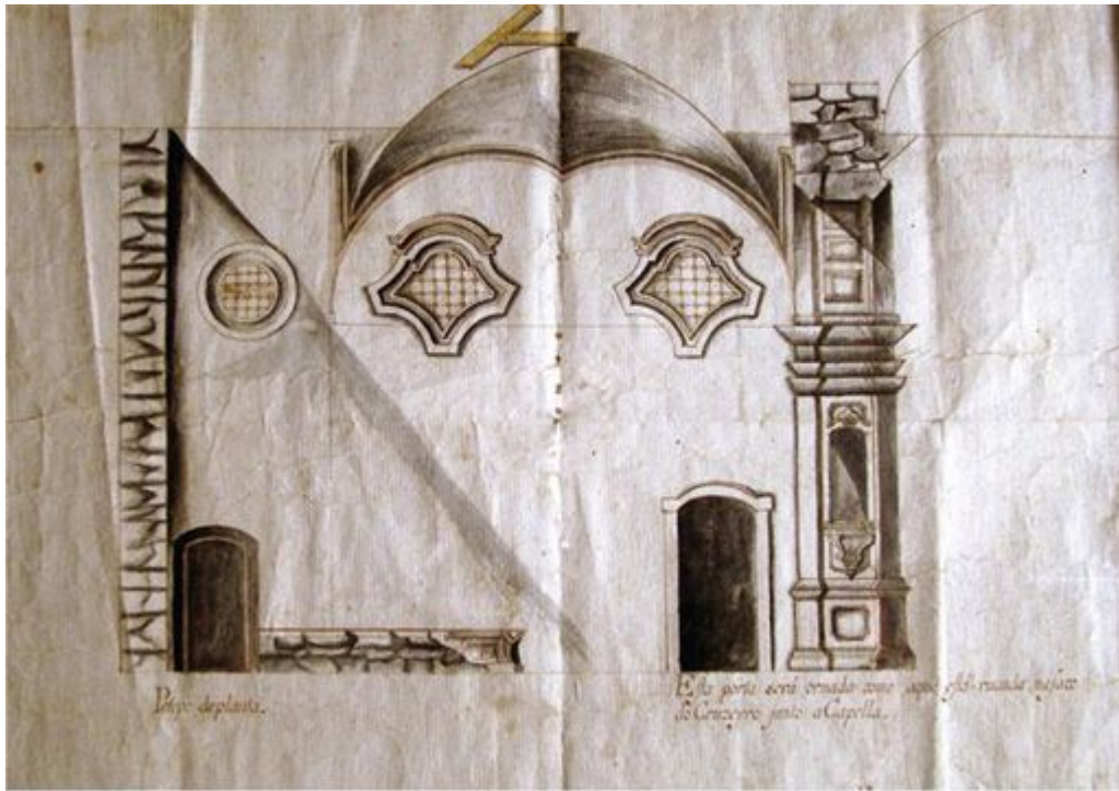
Corte original da capela-mor da Igreja de São Francisco de Assis em Ouro Preto. Desenho aquarelado, atribuído a Antônio Francisco Lisboa, o Aleijadinho, séc. XVIII. Acervo: Museu da Inconfidência . (Fotografia: Aldo Araújo)
