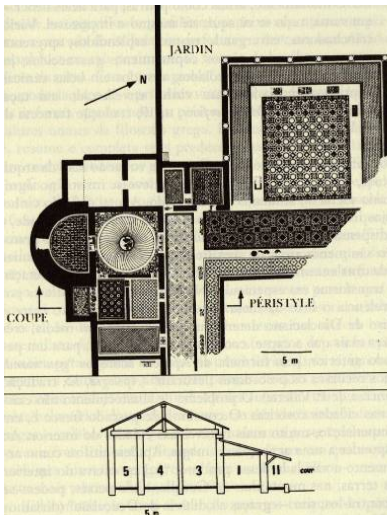
Figuras 13 e 14. Adrumeto, casa das máscaras (L. Foucher, La maison des masques, à Sousse, Túnis , 1965). Acima: um vasto triclinio, separado de um jardim por uma galeria, abre-se para o peristilo, a oeste. A êxedra de recepção, dotada de uma abside, localiza-se ao sul. Abaixo: corte reconstituído da ala sul passando sobre os aposentos situados a leste da êxedra (3-5) e sobre o pórtico meridional (1). [pág. 349]
