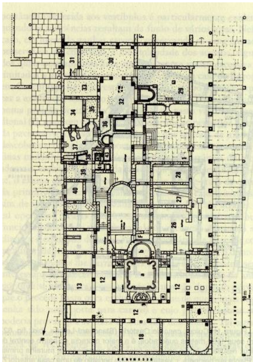
Figura 12. Cuicul, casa de Europa (Blanchard-Lemée, ibid. , fig. 49). Esta residência de 1366 metros quadrados nasceu da fusão de vários lotes (paredes de subdivisão I-J e F-F'). 1: vestibulo com porta tripartida; 12: pe-ristilo com pátio ocupado essencialmente por tanques (a, b, c) e jardineiras (d e d'); 13: triclínio; 18: triclínio ou êxada; 26: vestibulo; 27-8: lojas; 29-43: termas com latrinas em 29. [pág. 342]
