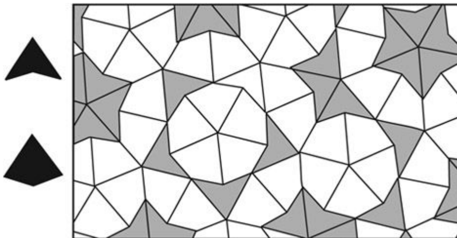
Figura 14. Usando dois tipos diferentes de azulejos, a pipa e o dardo, Roger Penrose foi capaz de cobrir esta superfície. Contudo, os azulejos de Penrose não possuem simetria translacional.
