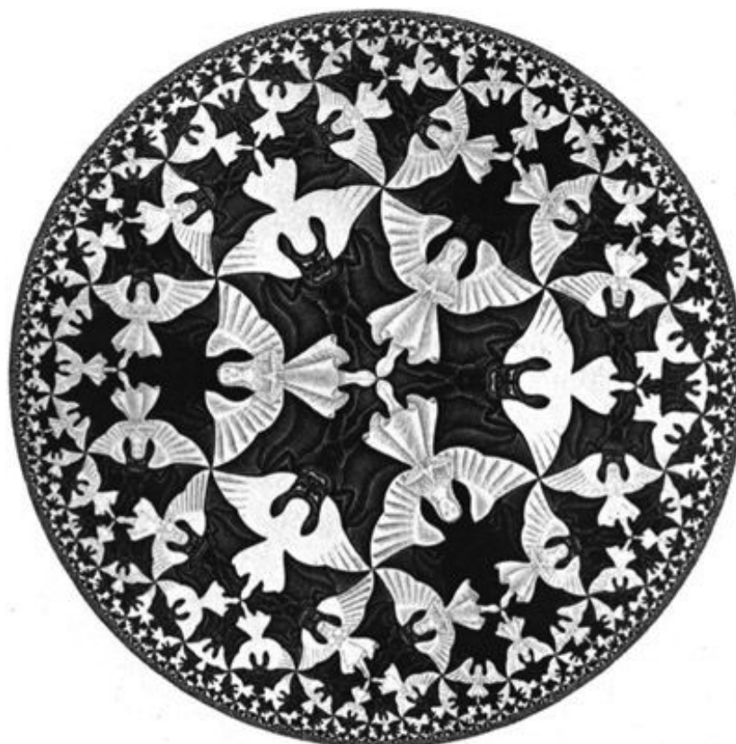
Figura 15. Limite circular IV, de Mauritz Escher, transmite um pouco da simetria das formas modulares.
