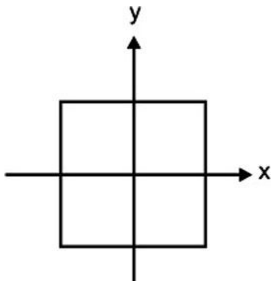
Figura 12. Um quadrado simples exibe a simetria rotacional e reflexiva.
