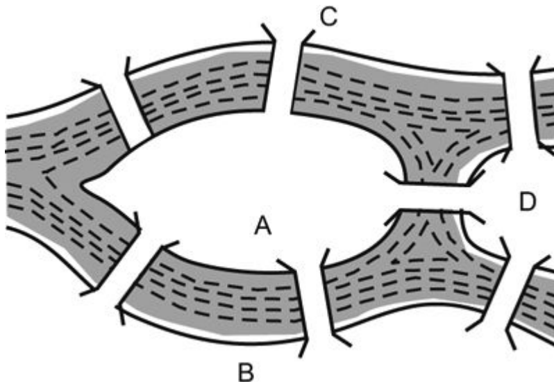
Figura 5. O rio Pregel divide a cidade de Königsberg em quatro partes separadas, A, B, C e D. Sete pontes ligam as várias partes da cidade, e um enigma local pergunta se é possível fazer um passeio de modo que cada ponte seja atravessada uma vez e somente uma vez.
