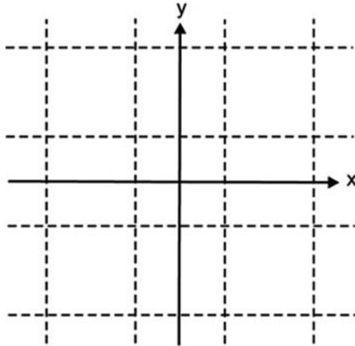
Figura 13. Uma superfície infinita, calçada com azulejos quadrados, exibe simetria rotacional e reflexiva, e além disso possui simetria translacional.
