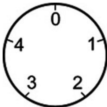
Figura 11. Na aritmética do relógio 5 a linha dos números foi cortada no cinco e dobrada sobre si mesma. O número 5 então coincide com o 0 e portanto é substituído por ele.
