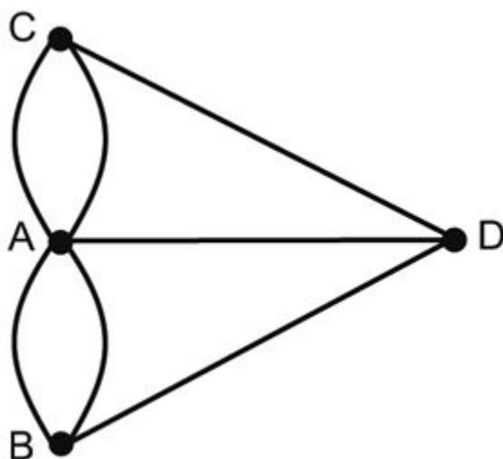
Figura 6. Uma representação simplificada das pontes de Königsberg.
