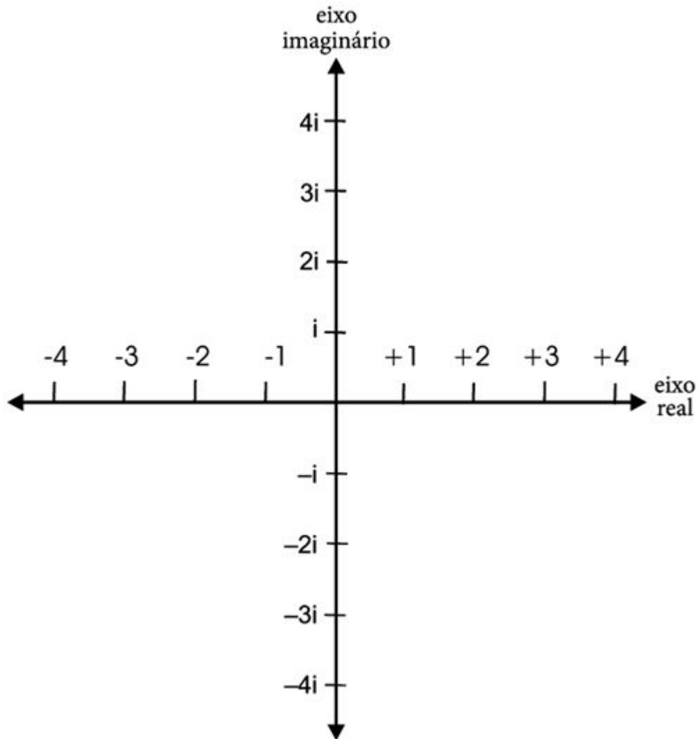
Figura 8. A introdução de um eixo para os números imaginários transforma a linha dos números num plano dos números. Qualquer combinação de números reais e imaginários tem uma posição no plano dos números.
