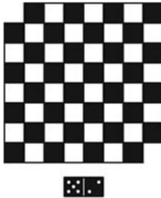
Figura 2. O problema do tabuleiro de xadrez mutilado.
