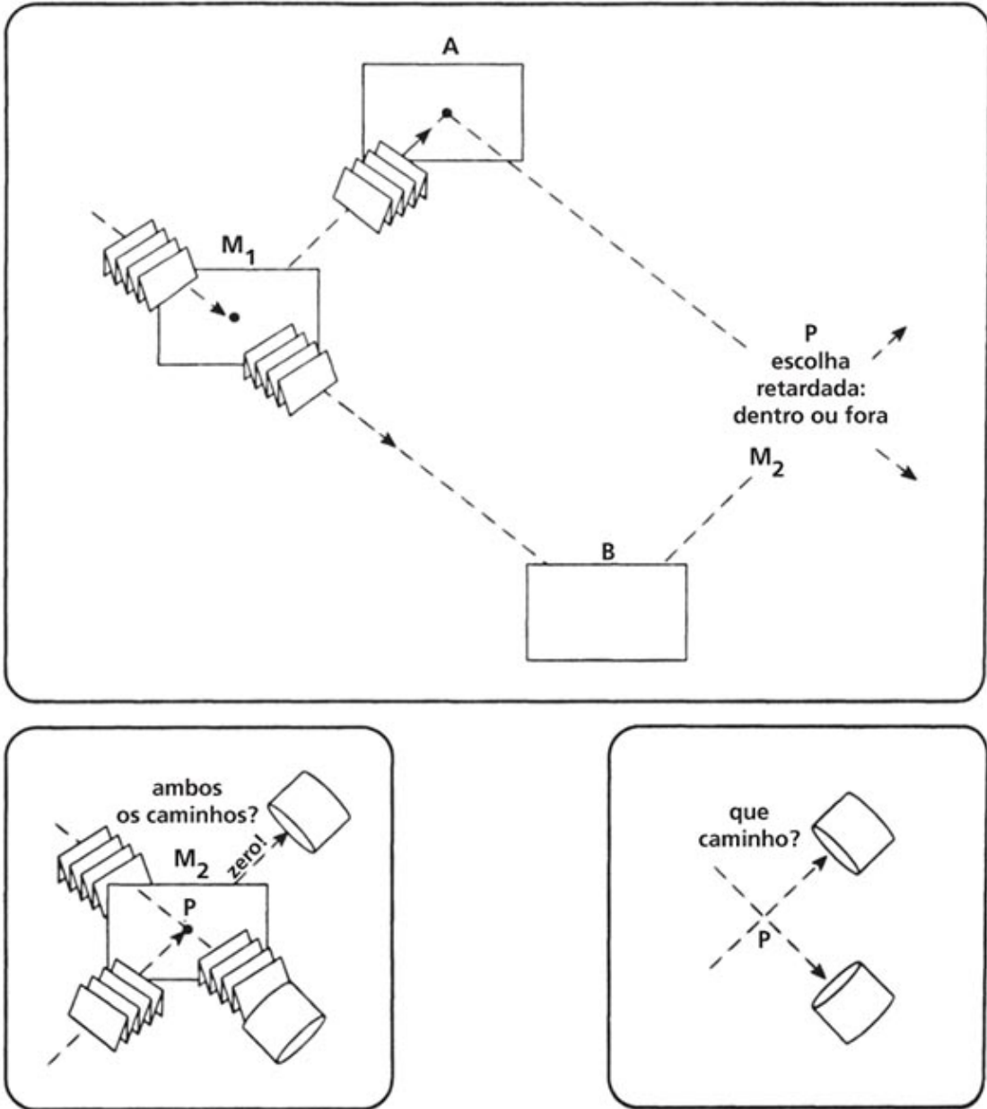
Figura 20. O experimento de escolha retardada. CANTO INFERIOR ESQUERDO: arranjo para se observar a natureza de onda do elétron. Um dos detectores jamais detecta quaisquer fótons, significando anulação devido à interferência de onda. O fóton deve ter se dividido e passado por ambos os caminhos ao mesmo tempo. CANTO INFERIOR DIREITO: arranjo para se observar a natureza de partícula do fóton. Ambos os detectores clicam – embora apenas um de cada vez – indicando qual o caminho tomado pelo fóton.
