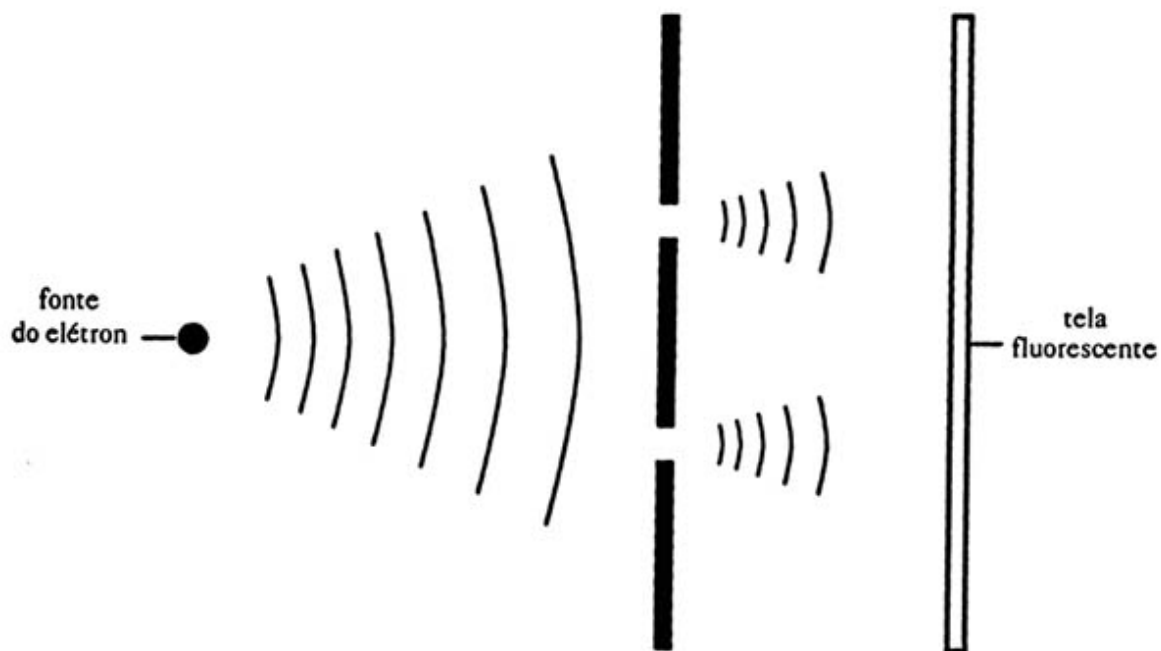
Figura 14. O experimento de fenda dupla com elétrons.
