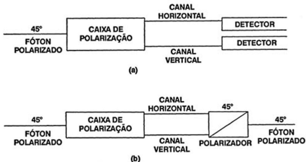
Figura 28. Experimentos com fótons polarizados a 45°.
