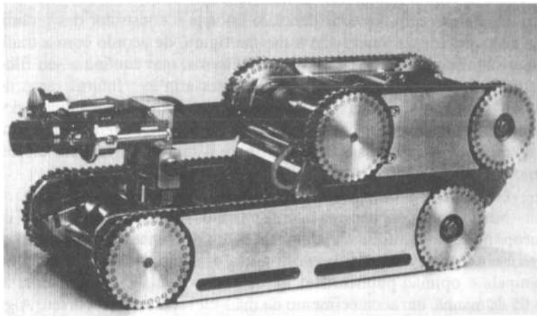
Robô Uruaut, construído por Rudolf Gantenbrink.
